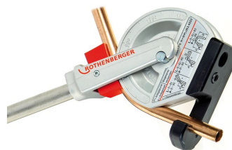
Rohrbiegezange "Robend H + W"
