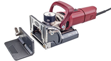
Nutfräse
