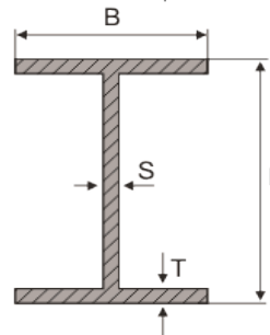
IPE-Profil (Beispiel)
