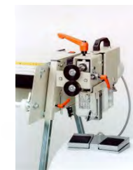
Zuschneidevorrichtung mit Sickenmaschine
