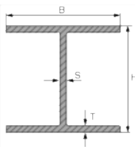
HEB-Profil (exemple)
